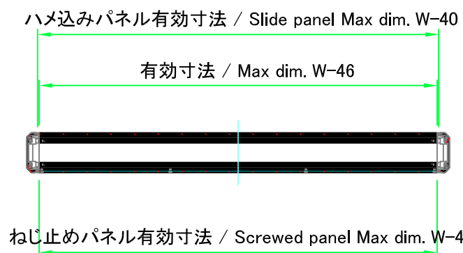
A-A ( 1 : 10 )
